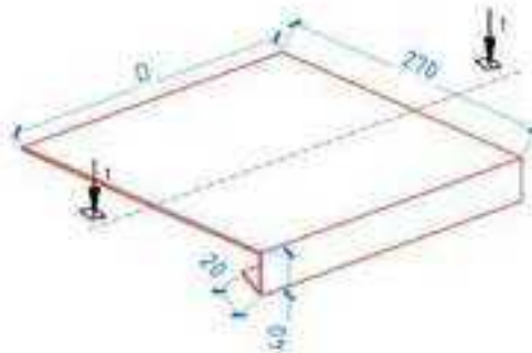
Отлив (поз.3) - схема изготовления
