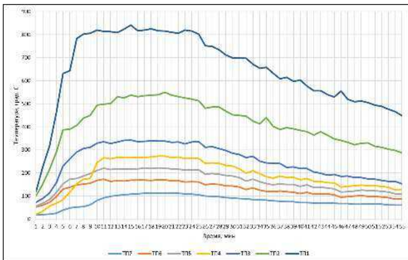
Рисунок 6. График изменения температур на термопарах T1-T7 при проведении испытания образца
