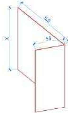
Элемент ППО (поз.5) – схема изготовления
