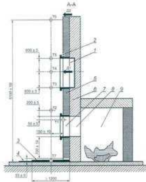
Рисунок 1 - Схема установки с образцом фасадной системы
