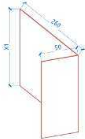
Элемент ППО - схема изготовления
